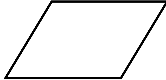
Input / Output
